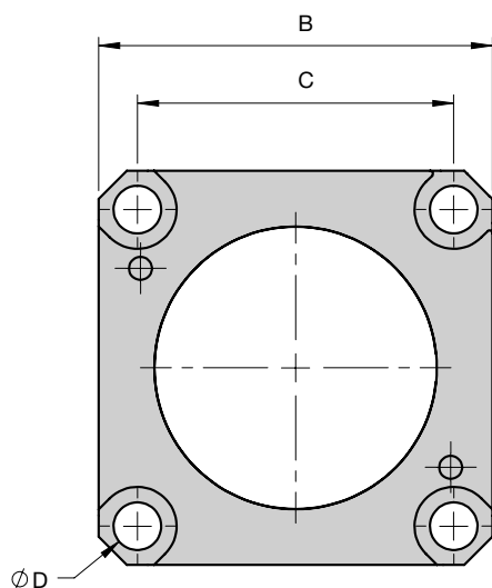
FCSC Halteflansch
