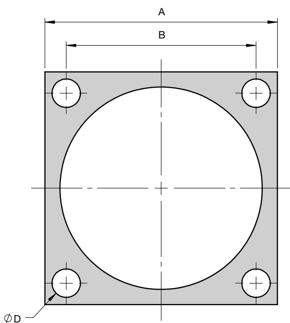
BFP Halteflansch
