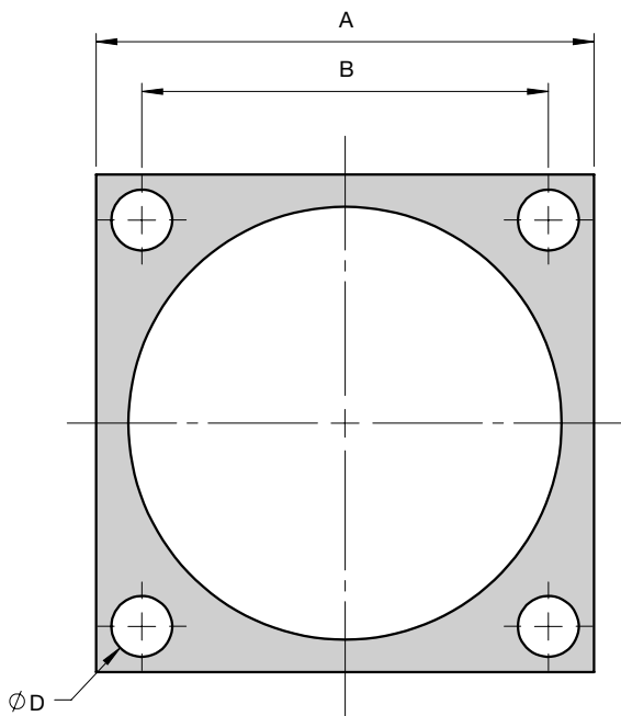
BFCU4 Halteflansch
