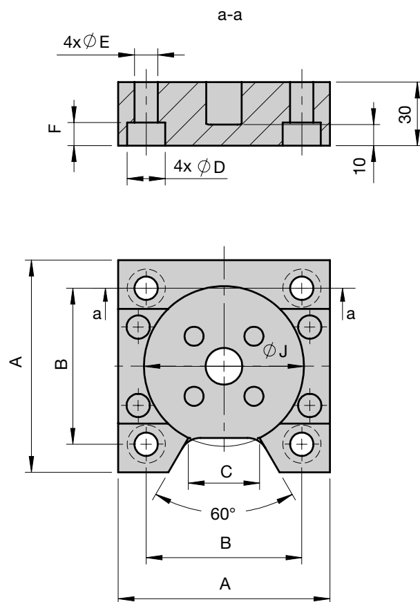
RM Halteflansch
