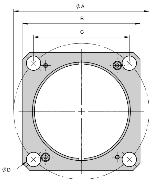
FK Halteflansch
