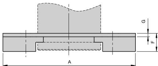
L Flange
