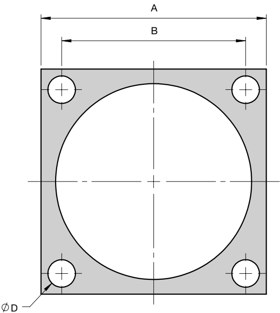
BFCU Flange
