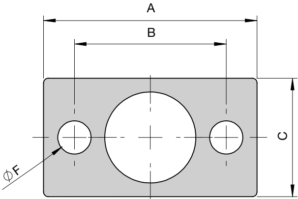
BF Flange
