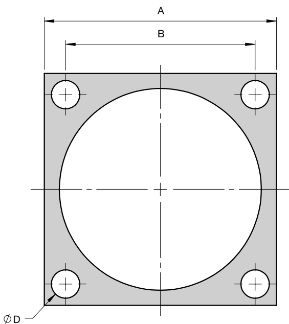
BFCU Flange
