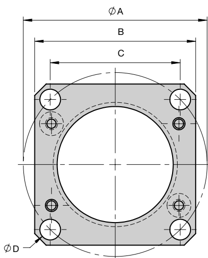
FCS Halteflansch
