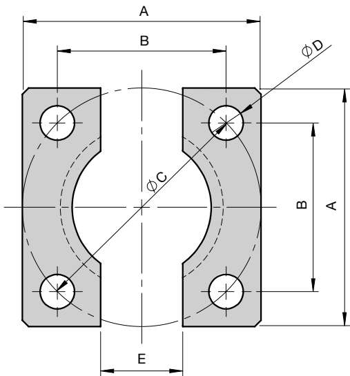
FFX Flange
