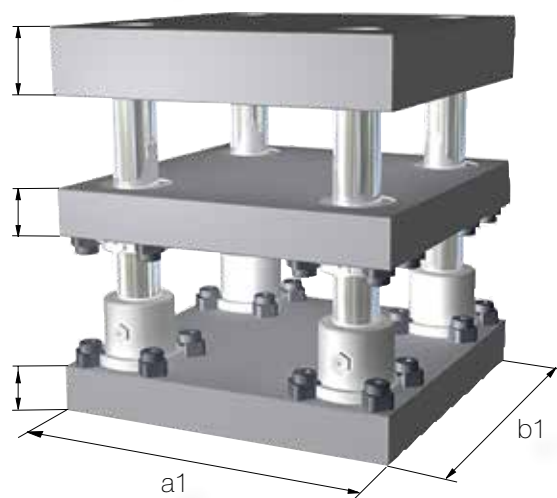
Zwischenplatte Intermediate plate
