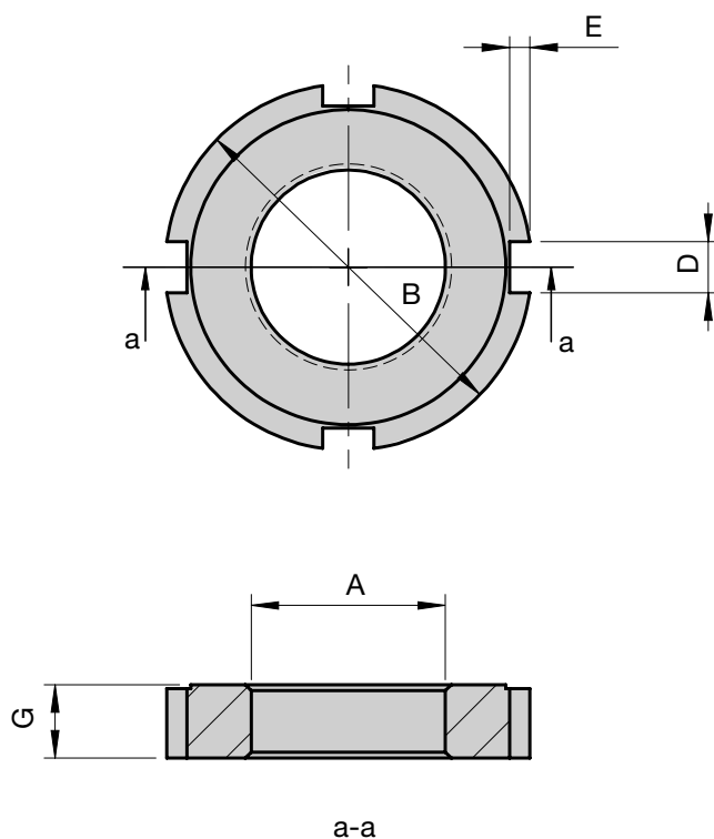
FRM Halteflansch
