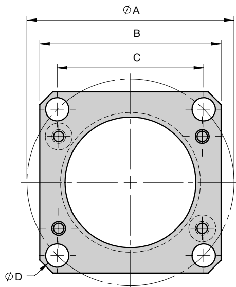
FCSX Flange
