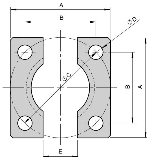
FFL Flange
