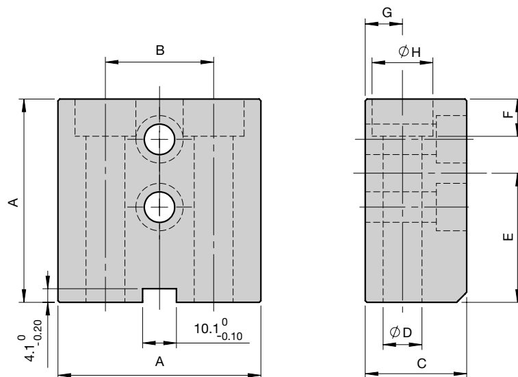
SA Halteflansch
