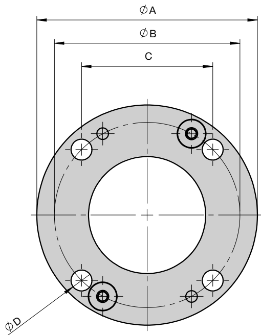
XFC Flange
