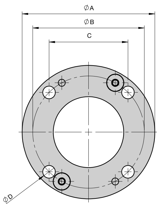
XFCJ Flange
