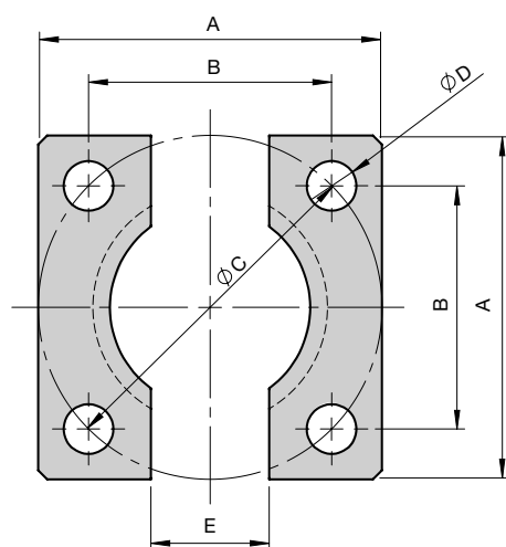
FFC Halteflansch
