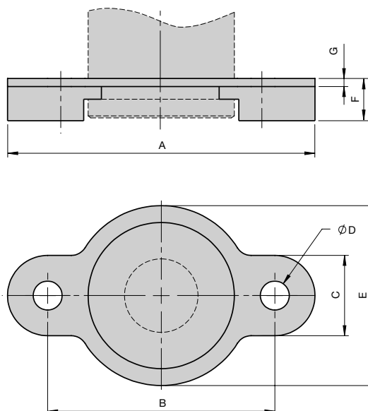
L Halteflansch
