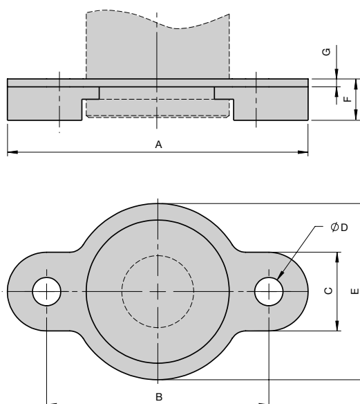
LX Halteflansch
