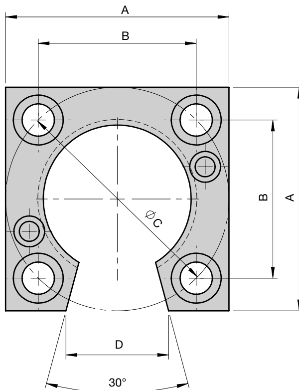
FSL Flange
