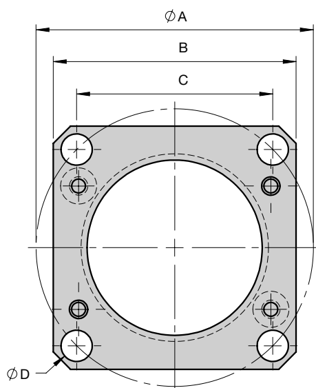
FCX Halteflansch
